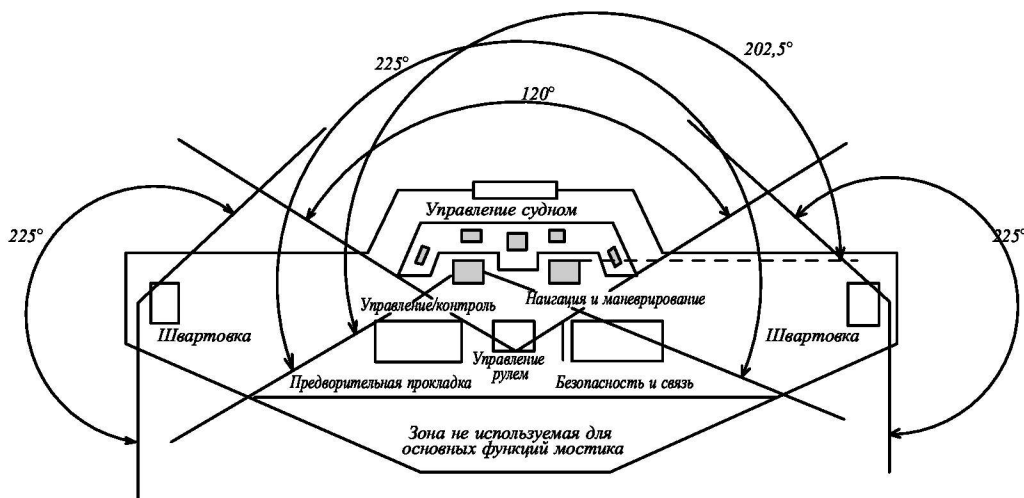
Рис. 2.5.17-1 Расположение рабочих постов и требуемые зоны видимости для них. Определение местоположения на бумажных картах — проход и место управления судном впереди
