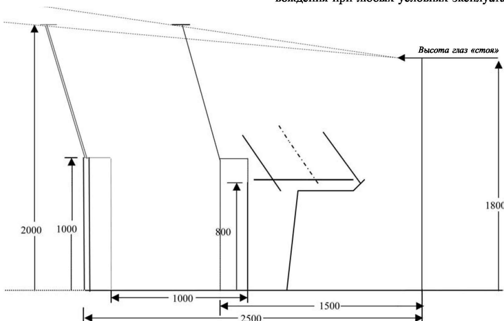
Рис. 2.6.3 При наклоне передних окон на угол 15° от вертикали угол обзора 5° выше горизонтали от уровня глаз стоящего человека, находящегося на высоте 1750 мм, может быть обеспечен на расстоянии 2600 мм от фронтальной стенки (лобовой переборки) с учетом наличия прохода шириной 1000 мм перед пультами рабочего поста
